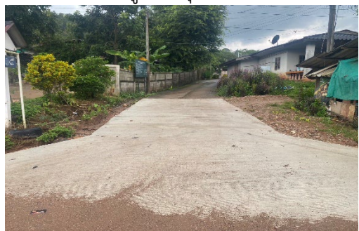
ก่อสร้างถนนคอนกรีตเสริมเหล็กเชื่อมถนนสายหลัก บ้านปางกอก หมู่ที่ 9 (จุดที่ 3) ซอย 5
